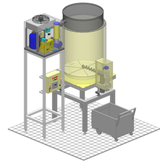
Silo AS 500 avec machine à glace
